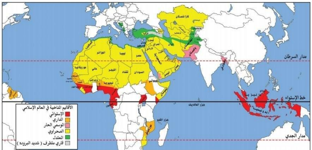
شكل (٣٠) خريطة الأقاليم المناخية في دول العالم الإسلامي
