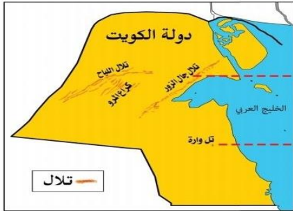
شكل (٢٦) تلال دولة الكويت
