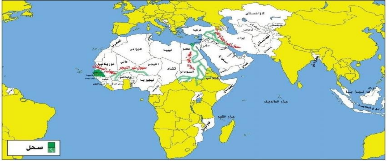
شكل (٢٧) خريطة لأهم السهول الفيضية في العالم الإسلامي
