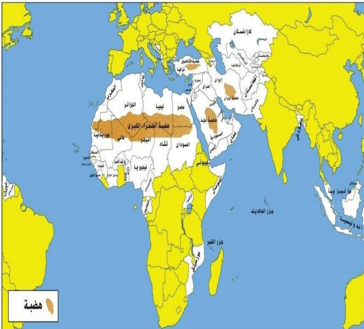
شكل (٢٤) أهم هضاب دول العالم الإسلامي
