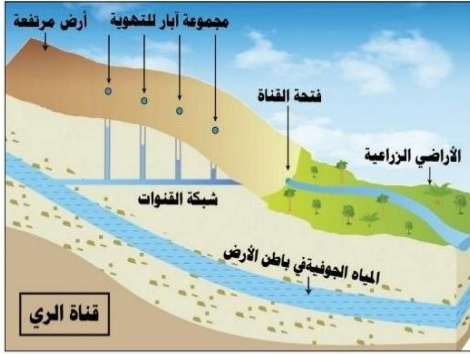
شكل (٥) النظام الذي تعمل به قناة الري
